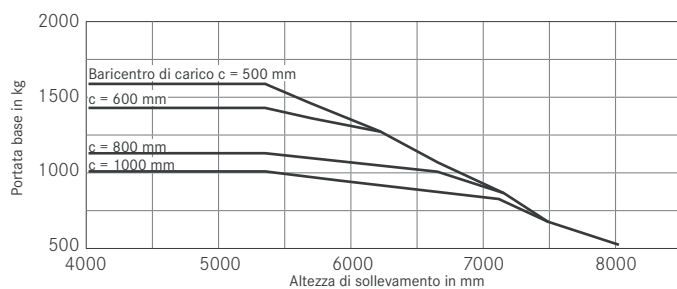
RX 70-16 Montante triplex Gommatura superelastiche
