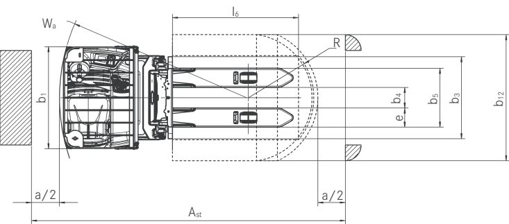
Vista dall'alto FXV
