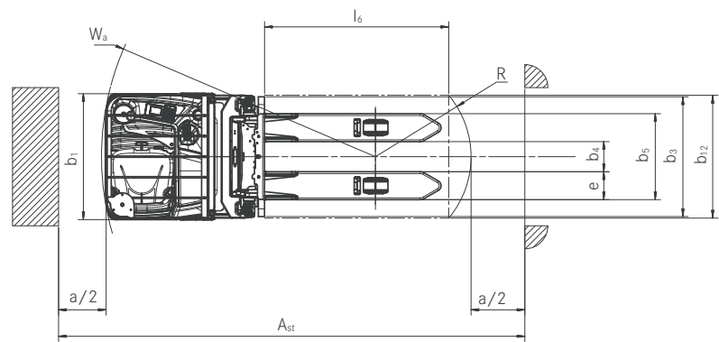
Vista dall'alto FXV N
