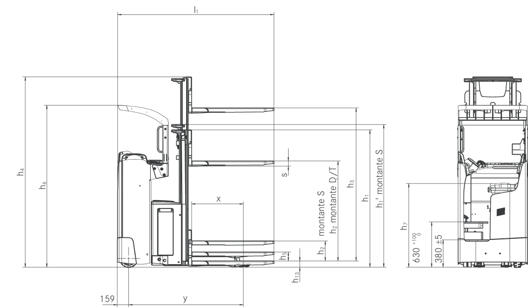
Vista laterale FXV
