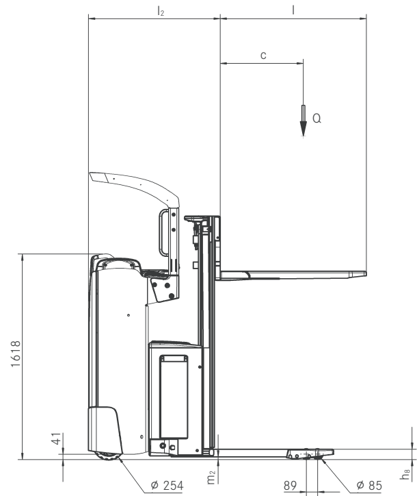
Vista laterale FXV
