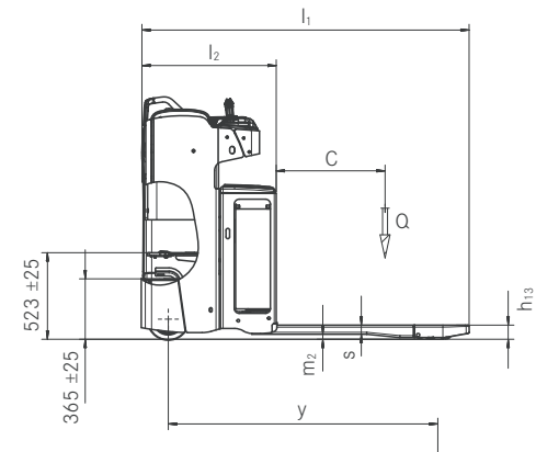
Vista laterale FXH N
