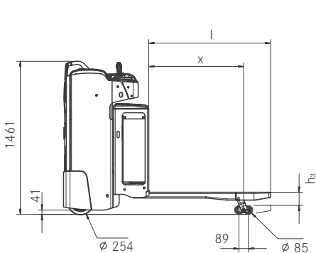
Vista laterale FXH N
