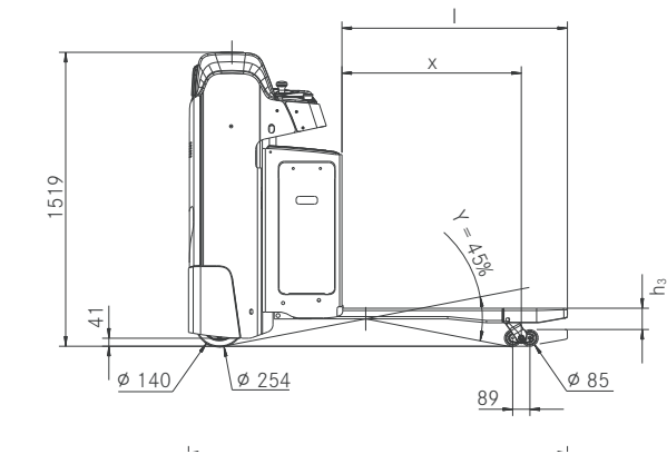
Vista laterale SXH con sollevamento iniziale attivato
