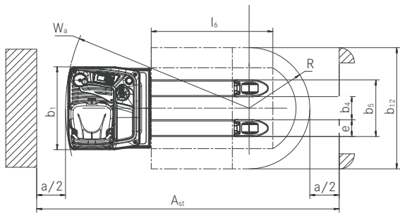
Vista dall'alto FXH N
